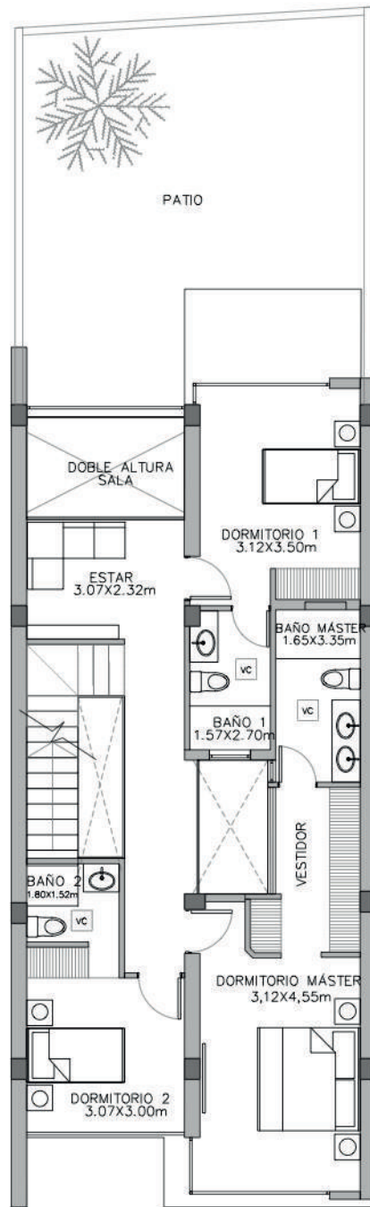
PLANTA ALTA
