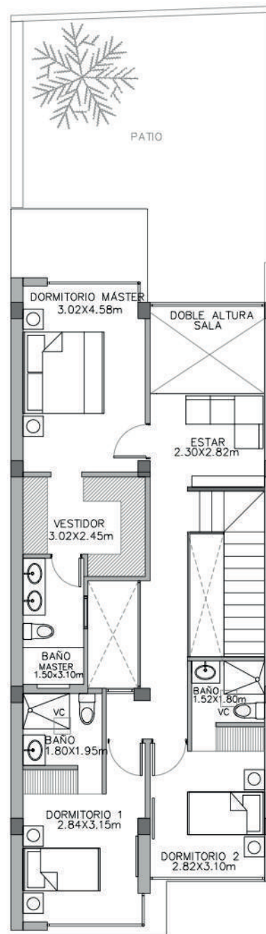
PLANTA ALTA
