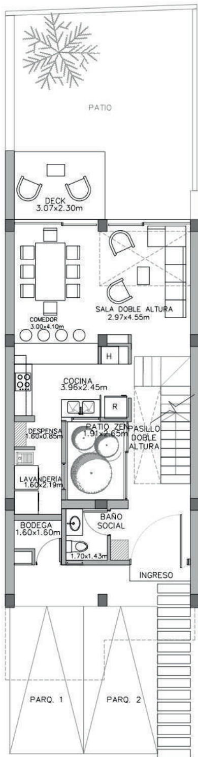
PLANTA BAJA
