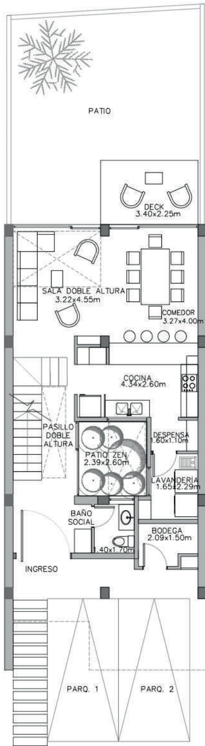
PLANTA BAJA
